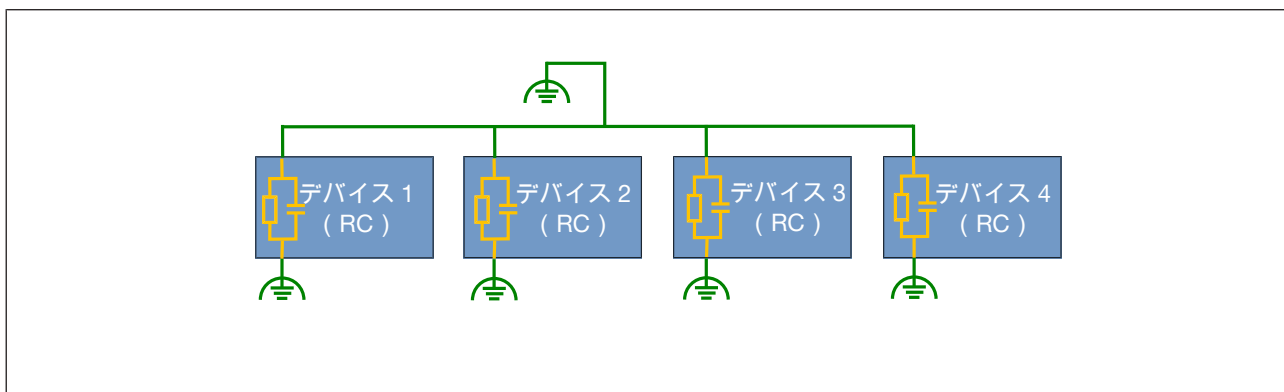
図 30: RCシールド
