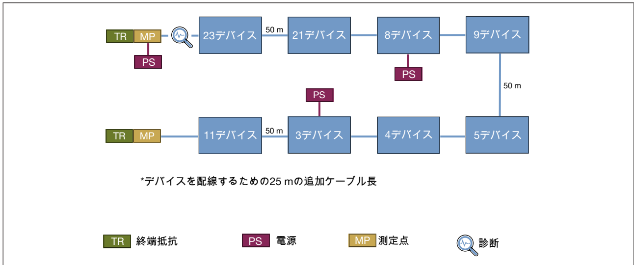
図 38: 250 kbit/s、84デバイス、ケーブル長175 m
