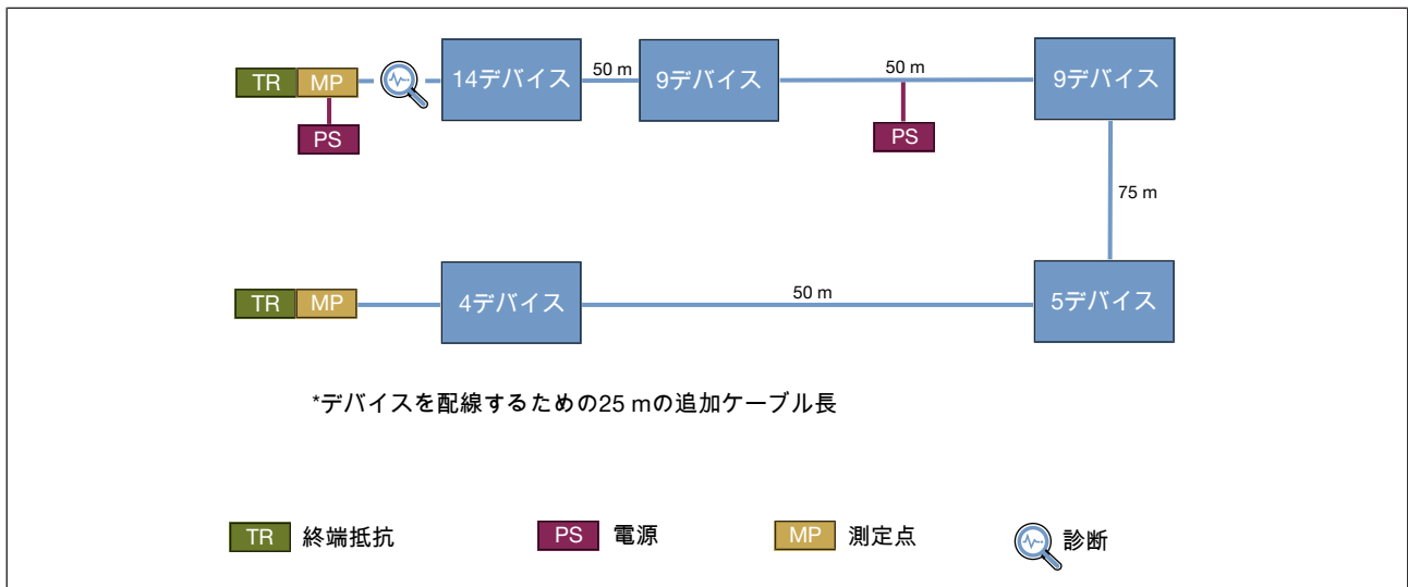
図 39: 250 kbit/s、41デバイス、ケーブル長250 m
