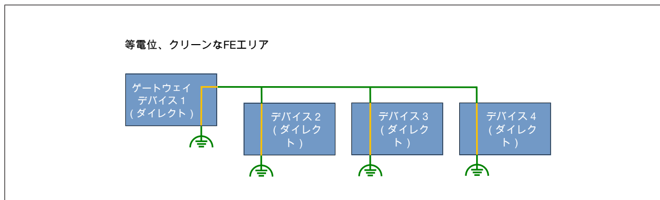
図 27: ダイレクトシールドデバイス
