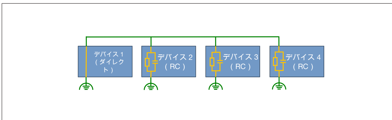
図 29: RCシールド
