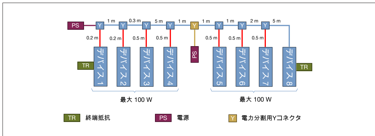
図 23: 追加の電源
