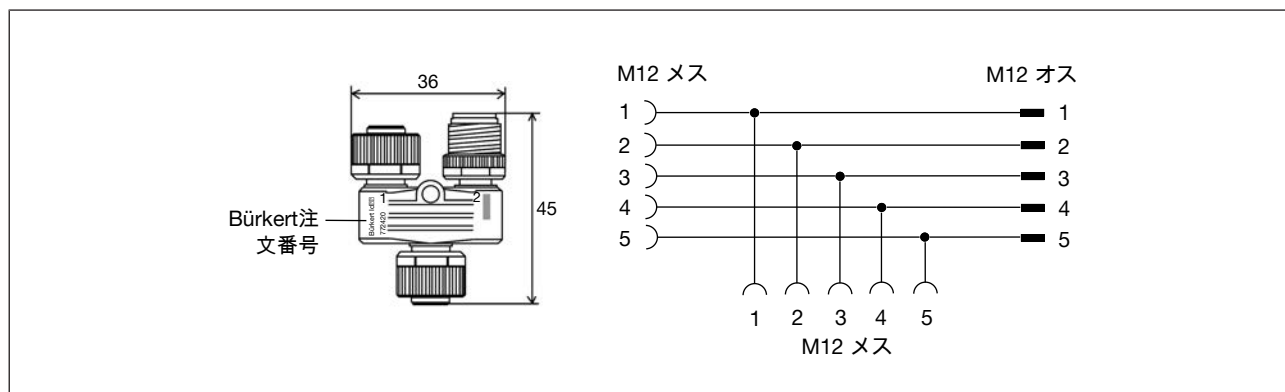
図 2: Yコネクタ
