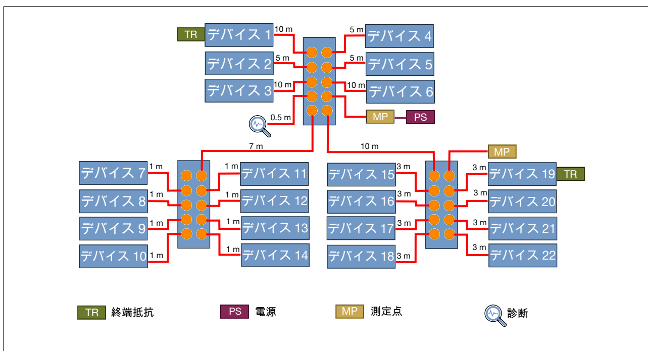
図 43: ジャンクションボックスを備えたツリートポロジ
