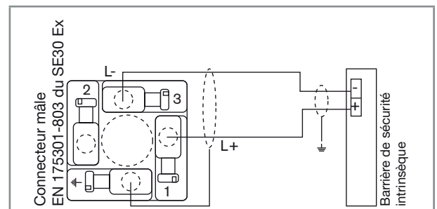
Fig. 5: Raccordement du SE30 Ex à une barrière de sécurité intrinsèque
