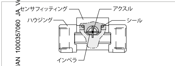
図 2: ねじ接続S030の断面
