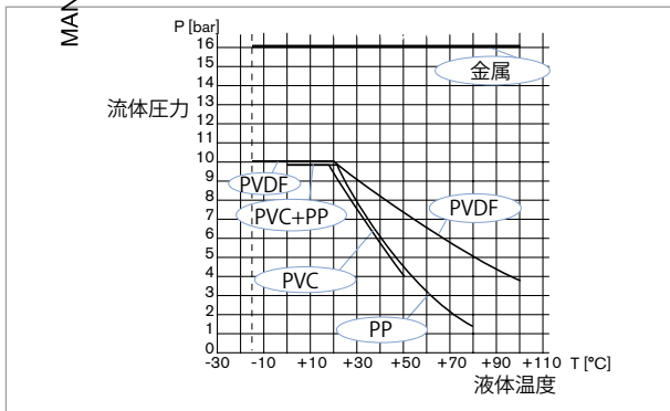
図 1: ねじ接続S030自体に対する液体の圧力対温度依存曲線
