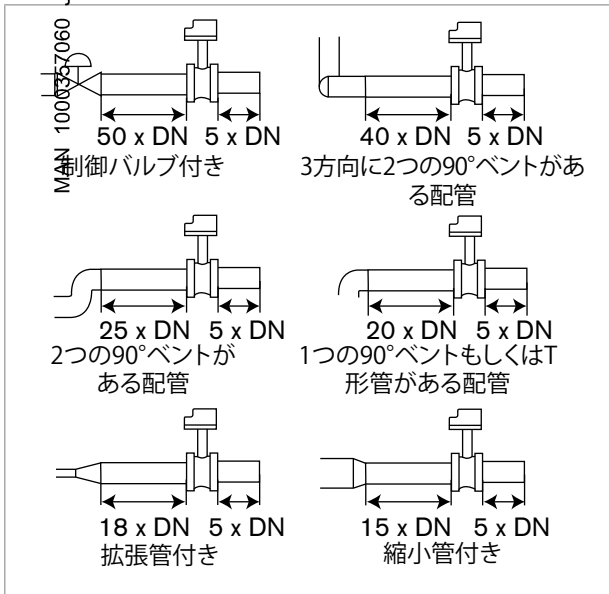
図 3: 配管の構造に応じた最低流入・流出距離距離
