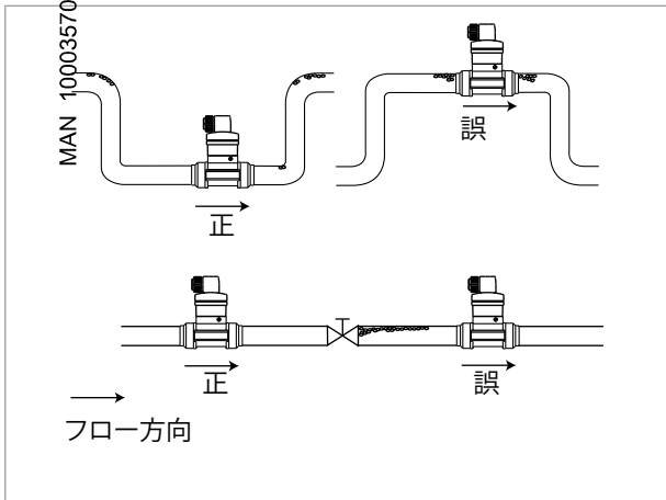
図 4: 取付に関する補足推奨事項
