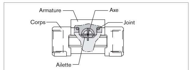
Fig. 2 : Vue en coupe d'un raccord S030
