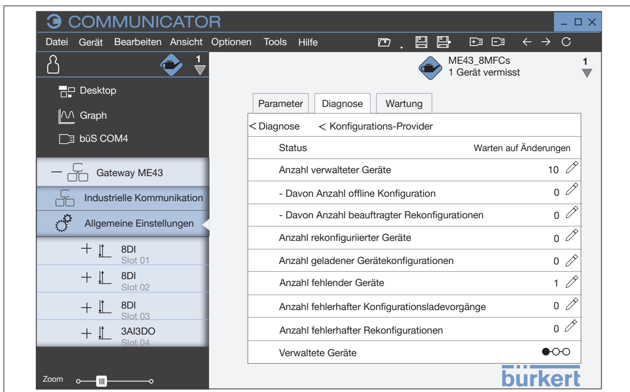
Bild 5: Detailsicht Diagnose für Konfigurations-Provider
