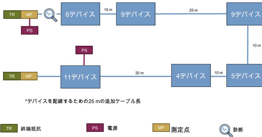
図 37: 500 kbit/s、44デバイス、ケーブル長100 m
