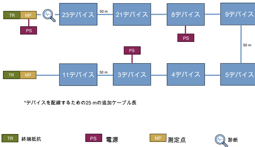
図 38: 250 kbit/s、84デバイス、ケーブル長175 m
