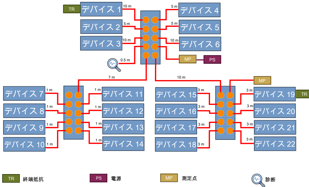
図 43: ジャンクションボックスを備えたツリートポロジ
