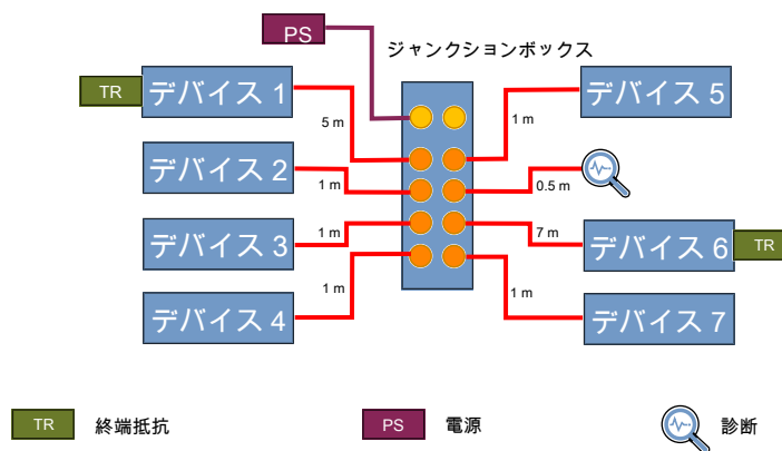
図 24: ジャンクションボックス付きネットワーク
