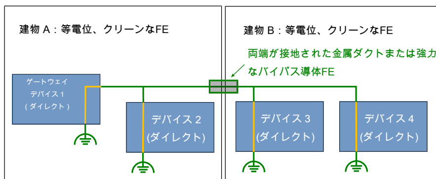
図 28: ダイレクトシールドデバイス、2つの建物
