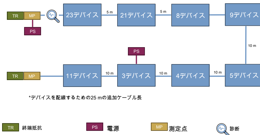
図 36: 500 kbit/s、84デバイス、ケーブル長75 m
