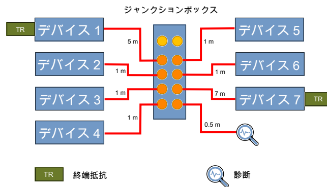
図 19: ジャンクションボックス付きネットワーク
