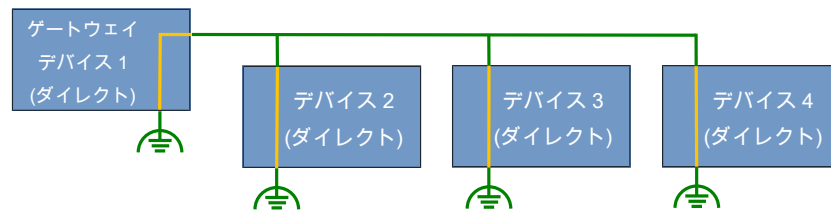
図 27: ダイレクトシールドデバイス
