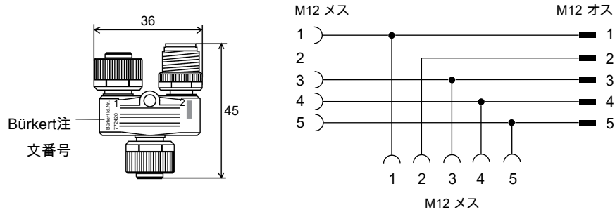
図 3: 電力分割用Yコネクタ
