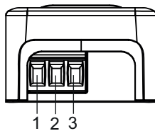
Abb. 9: Anschlussmöglichkeit für die Industrial-Ethernet-Variante
