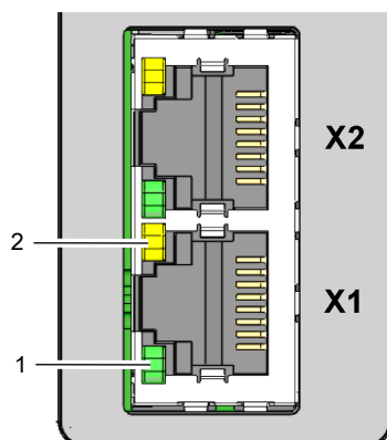
Abb. 5: Lage und Beschreibung der LEDs einer RJ45-Buchse
