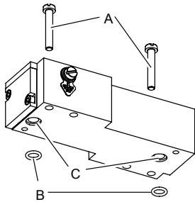
Fig. 6: Raccordement à bride avec vis et joints toriques
