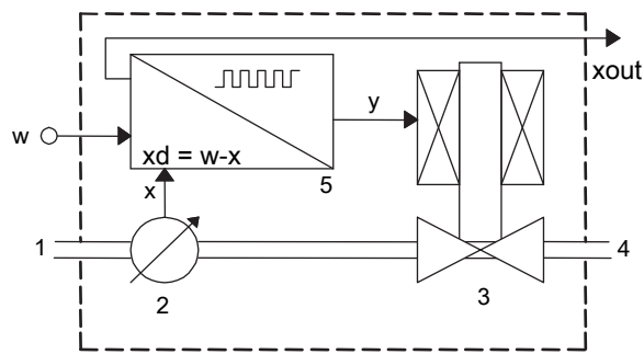
Fig. 9: Diagramme fonctionnel du MFC avec vanne de régulation
