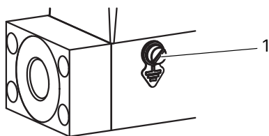
Fig. 7: Emplacement de la vis M4 pour le raccordement de la terre fonctionnelle
