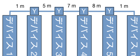
図 15: スタブラインのないYコネクタを備えたネットワーク
