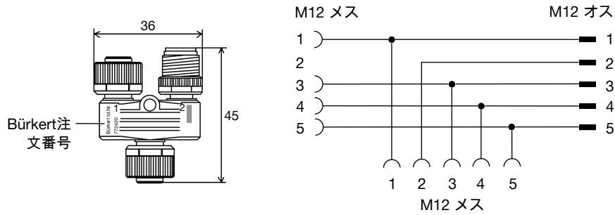
図 3: 電力分割用Yコネクタ
