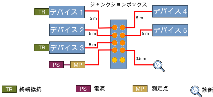
図 42: ジャンクションボックスを備えたスタートポロジ
