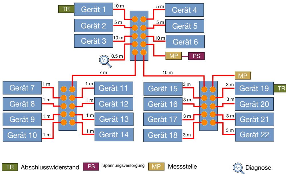
Abb. 43: Baumtopologie mit Verteilerdose
