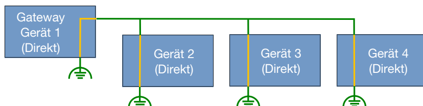
Abb. 27: Direkt geschirmtes Gerät
