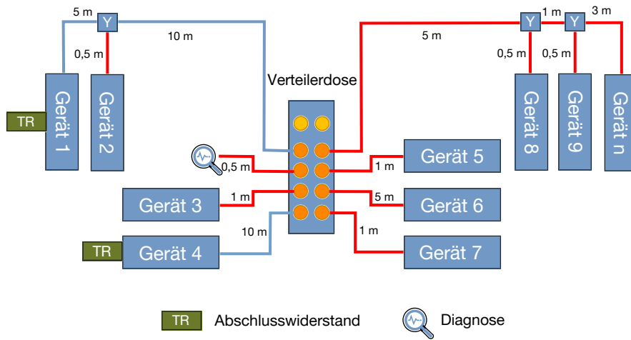
Abb. 21: Gemischte Netzwerke
