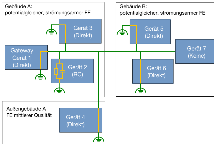
Abb. 33: Ursprüngliches Netzwerk
