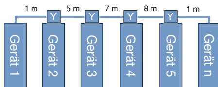
Abb. 15: Netzwerk mit Y-Steckverbindern ohne Stichleitungen
