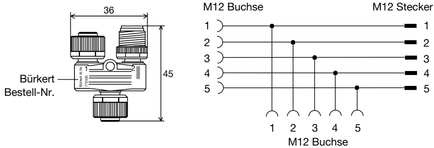
Abb. 2: Y-Steckverbinder
