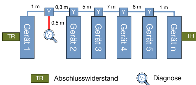
Abb. 20: Netzwerk mit Y-Steckverbindern
