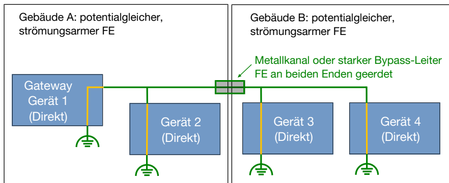
Abb. 28: Direkt abgeschirmtes Gerät, 2 Gebäude
