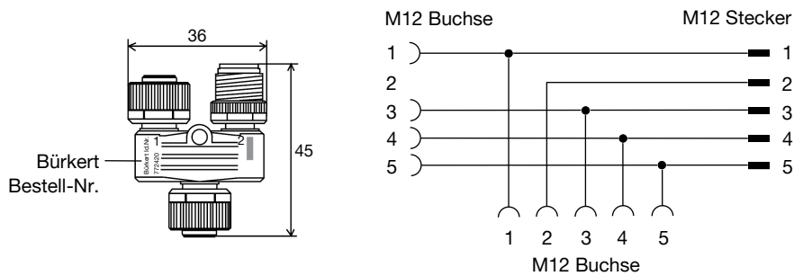
Abb. 3: Y-Steckverbinder mit Stromunterbrechung
