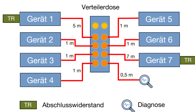
Abb. 19: Netzwerk mit einer Verteilerdose
