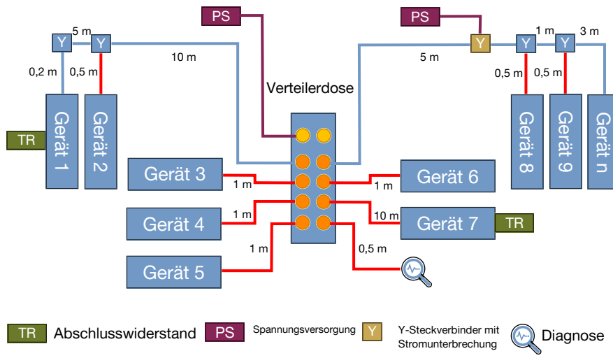
Abb. 26: Gemischte Netzwerke
