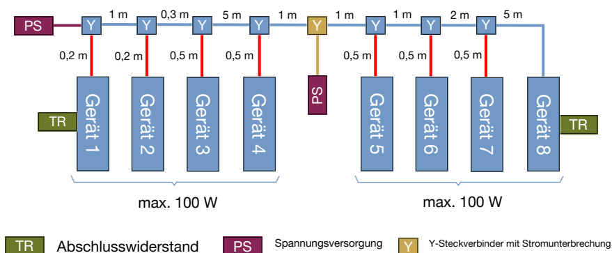
Abb. 23: Zusätzliches Netzteil
