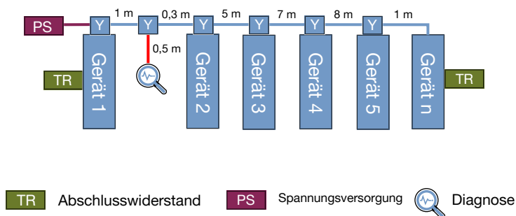
Abb. 25: Netzwerk mit Y-Steckverbindern
