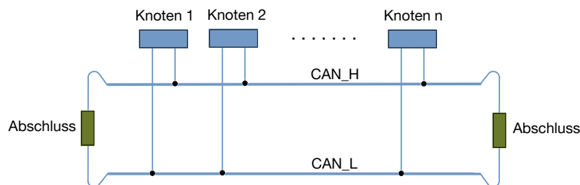
Abb. 18: Abschlusswiderstände
