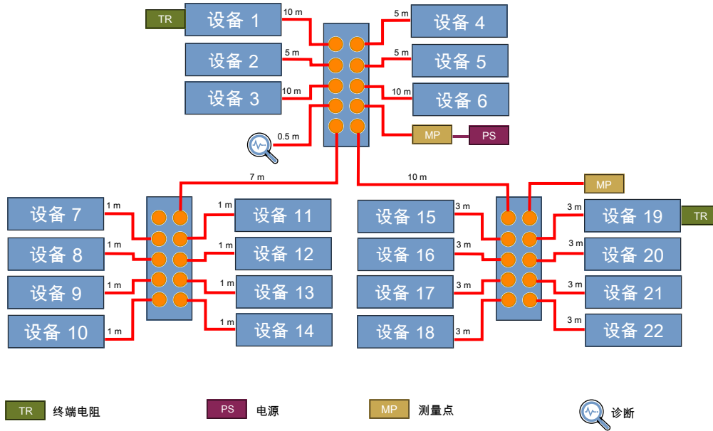
图 43: 带配电箱的树形拓扑
