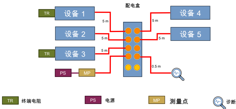
图 42: 带配电盒的星形拓扑
