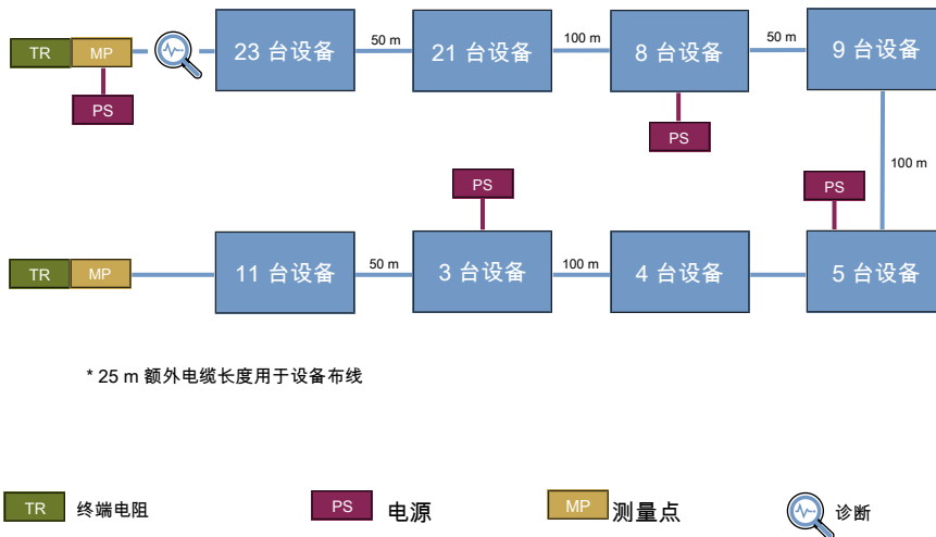
图 40: 125 kbit/s , 84 台设备 , 电缆长度 475 m
