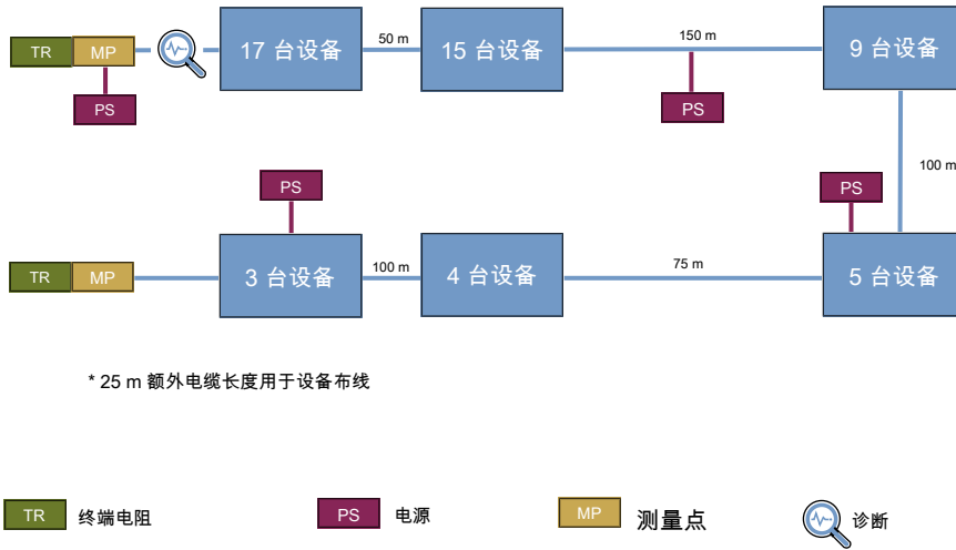
图 41: 125 kbit/s , 53 台设备 , 电缆长度 500 m
