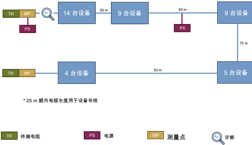
图 39: 250 kbit/s , 41 台设备 , 电缆长度 250 m
