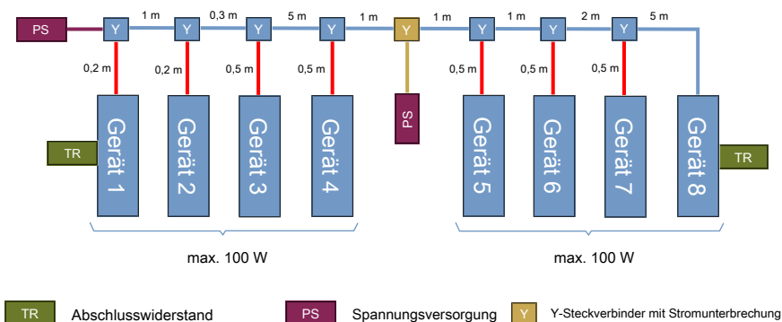
Abb. 23: Zusätzliches Netzteil
