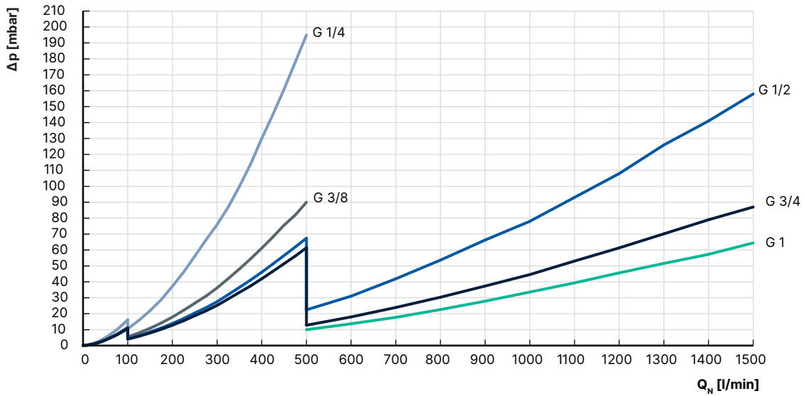
图 12: MFM 压力损失图
