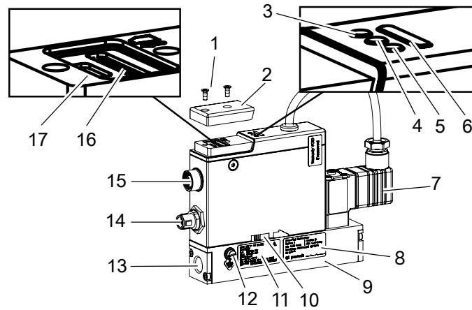
Fig. 6: Exemple de variante MFC Ethernet industriel
