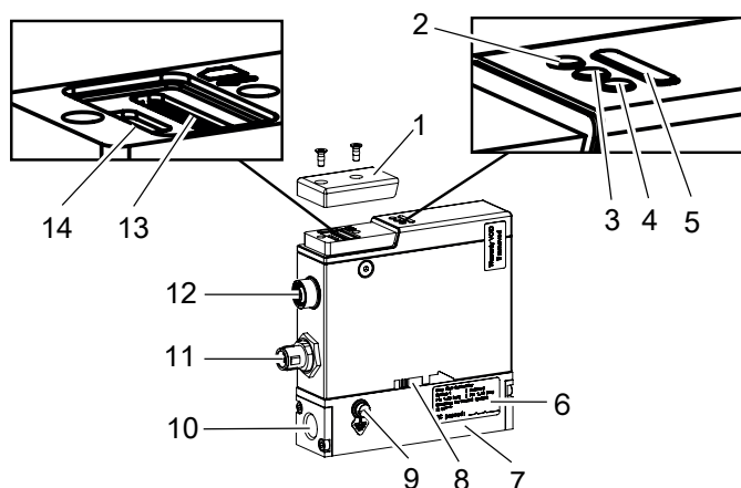
Fig. 3: Exemple de variante MFM PROFIBUS
