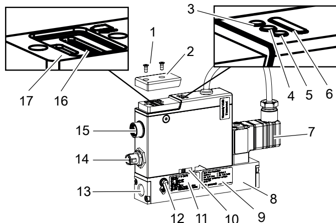
Fig. 7: Exemple de variante MFC PROFIBUS
