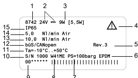
Fig. 9: Exemple d'étiquette d'identification Type 8742
