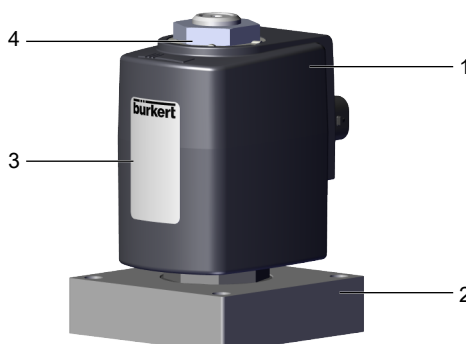
Fig. 2: Type 6020, variante à bride (exemple : FK15)
