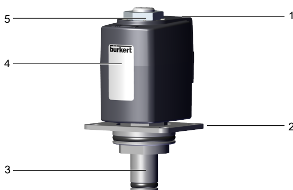
Fig. 1: Type 6020, variante à cartouche (exemple : FC17)
