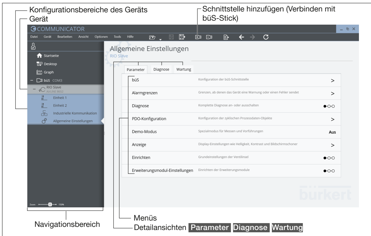
Bild 12: Beispiel einer Bedienoberfläche der Software Bürkert Communicator
