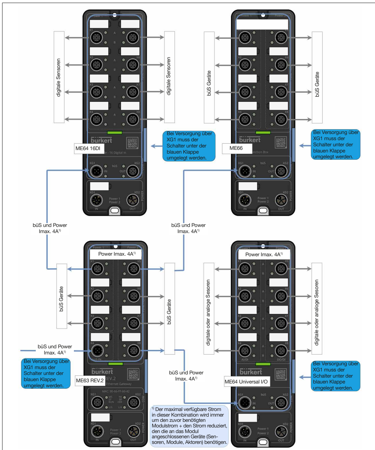
Bild 10: Beispiel für die Stromversorgung über bÜS
