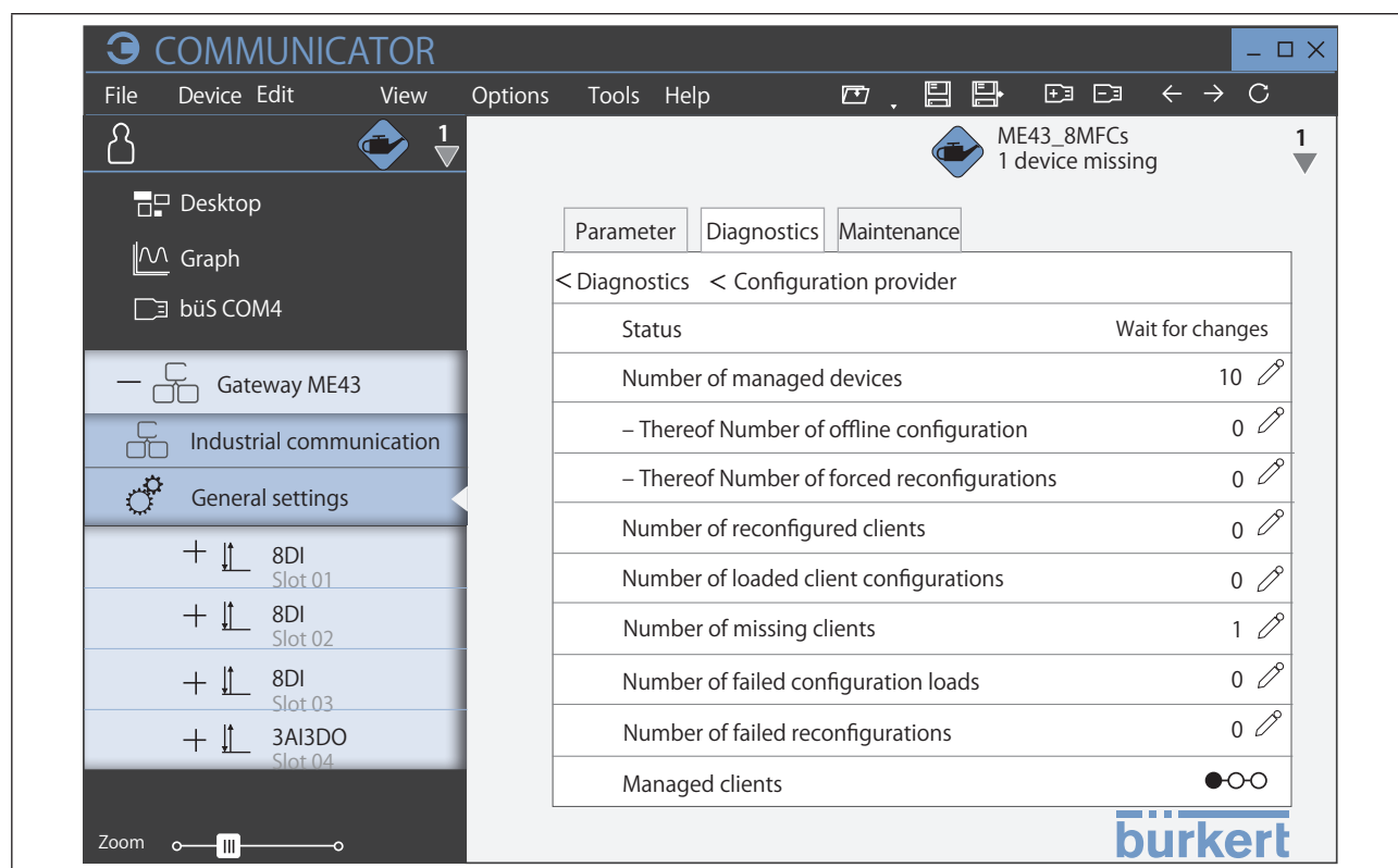
挿図 5: 構成プロバイダの診断の詳細ビュー
