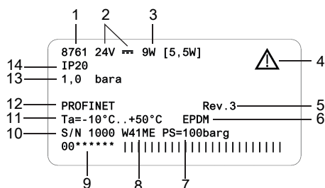
Fig. 1: Exemple d'une étiquette d'identification Type 8761
