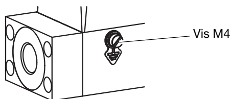
Fig. 11: Emplacement de la vis M4 pour le raccordement de la terre fonctionnelle
