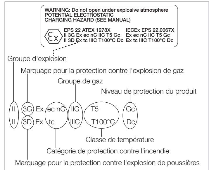
Fig. 2: Étiquette pour les zones Ex.
