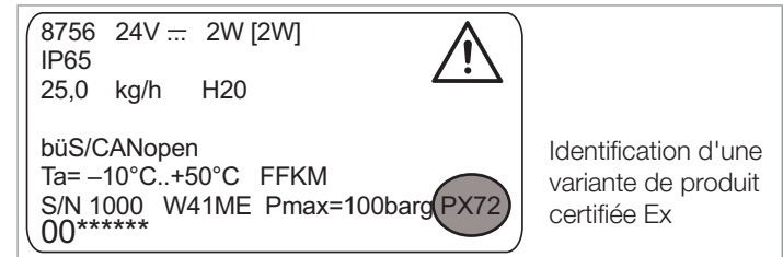
Fig. 1: Emplacement de la clé variable PX72 sur l'étiquette d'identification
