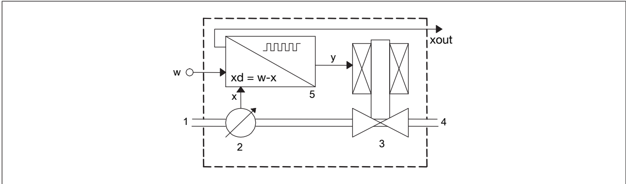
図 14: 比例バルブ付きMFCの機能図
