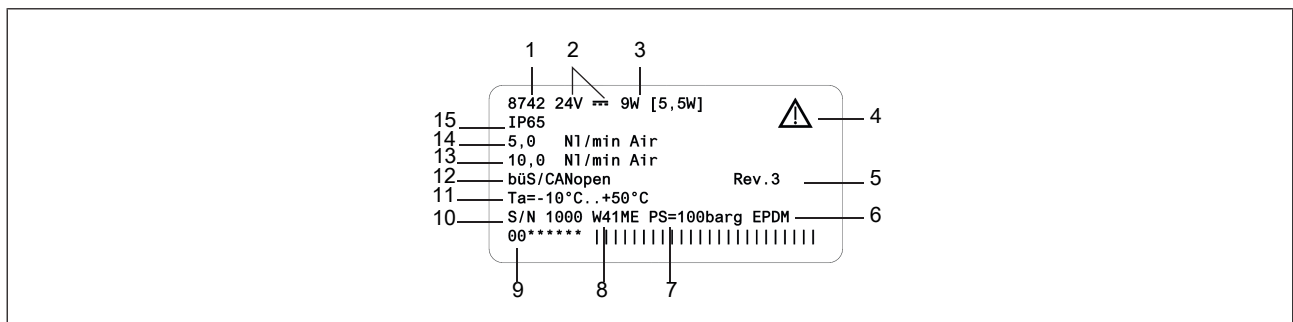
図 1: タイプ8742の銘板例
