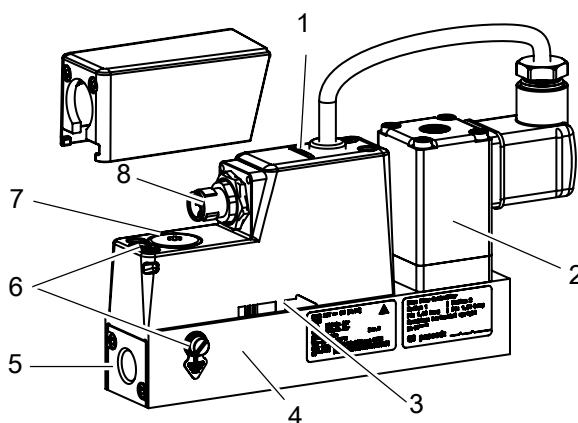
Fig. 8: Exemple de variante MFC bus/ CANopen
