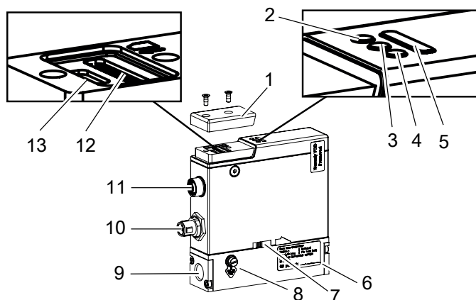
Fig. 3: Exemple de variante MFM PROFIBUS
