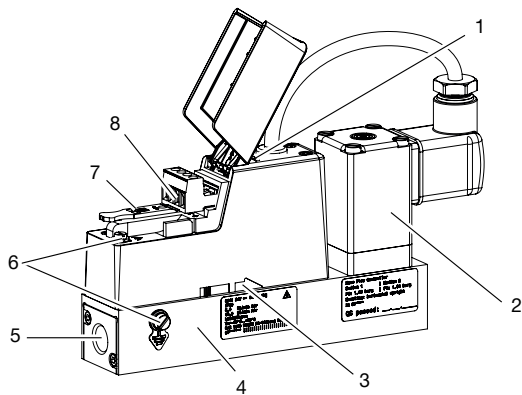
Esempio di una variante MFC con valvola proporzionale
