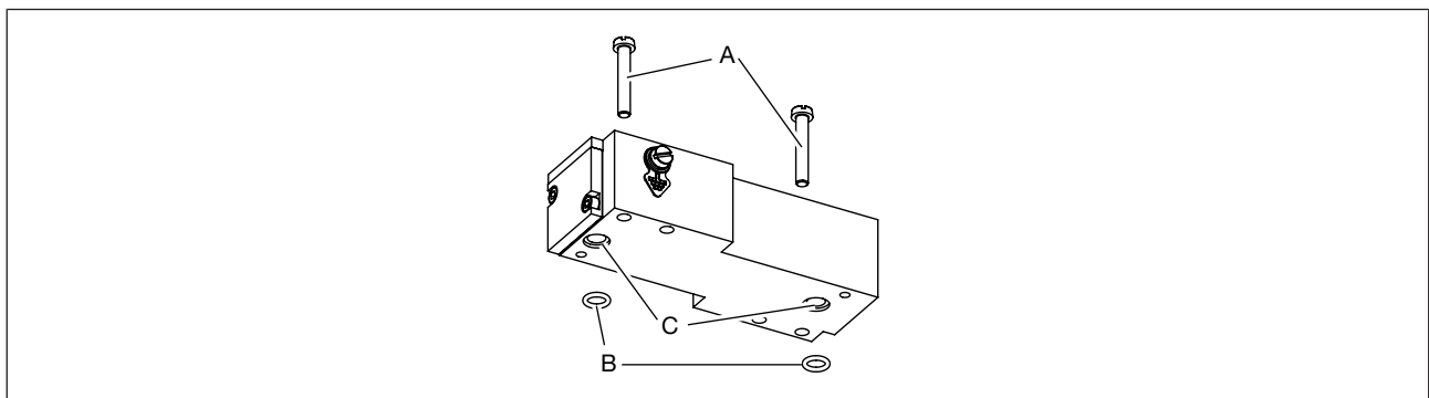
Abb. 11: Collegamento flangia con viti e guarnizione O-ring
