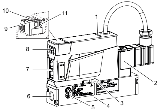
Esempio di una variante MFC con valvola proporzionale
