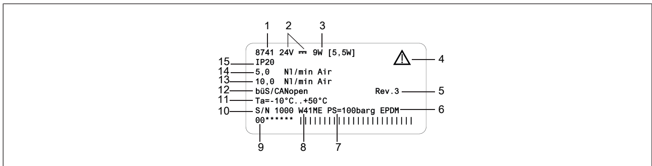
图 1: 8741 型铭牌示例
