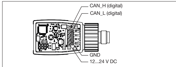
Bild 2: Anschluss Klemmleiste
