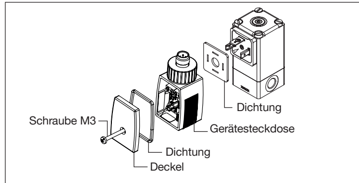
Bild 5: Montage der Ansteuerelektronik an das Ventil
