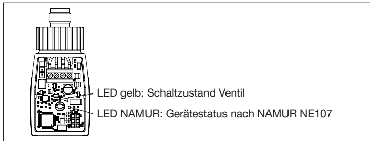
Bild 6: LED-Anzeige der Ansteuerelektronik ohne Bedieneinheit
