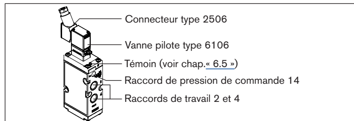
Fig. 1 : Ensemble de vanne type 6516 /6517 (exemple, type 6517)
