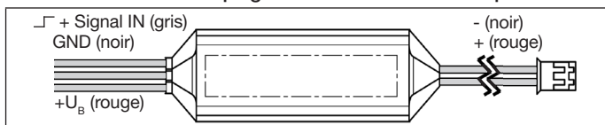
Fig. 1 : Raccordement de la vanne
