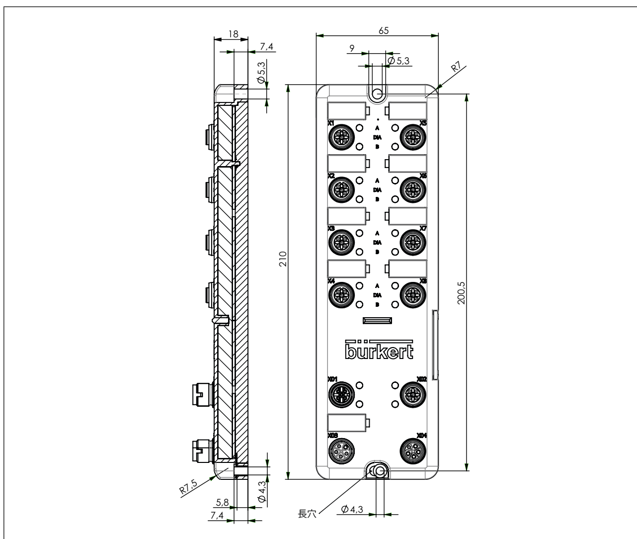
挿図 2: 寸法 I/O モジュール FieldConnect タイプ ME64
