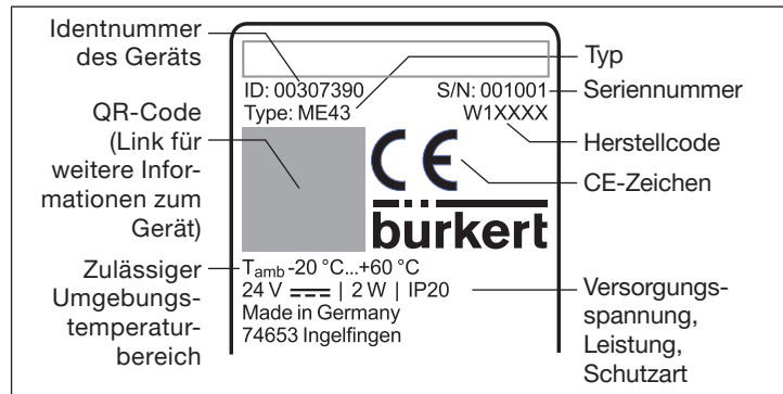
Bild 1: Beschreibung Typschild und Gerätebeschriftung
