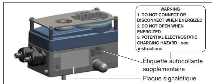
Fig. 1 : Disposition des étiquettes autocollantes pour la zone présentant des risques d'explosion, étiquette autocollante supplémentaire
