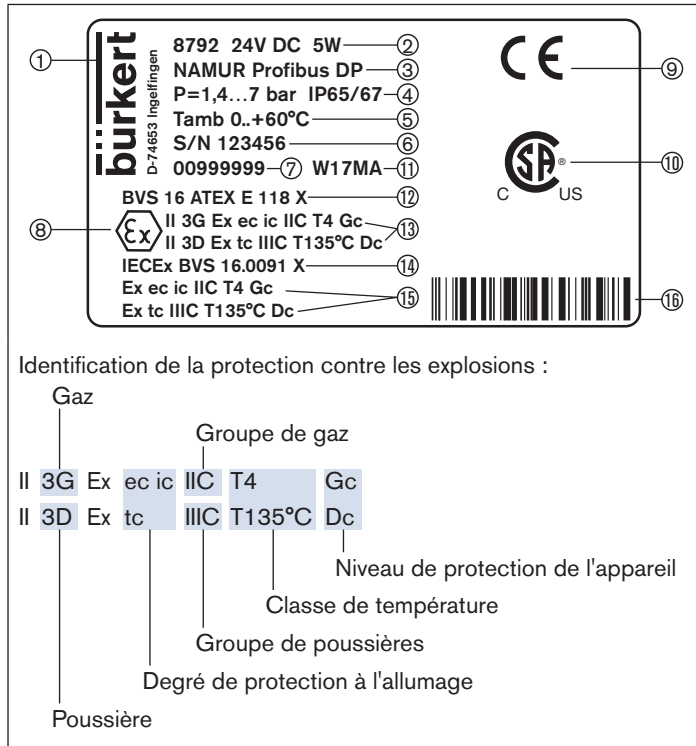
Fig. 2 : Plaque signalétique (exemple) d'un appareil avec homologation Ex
