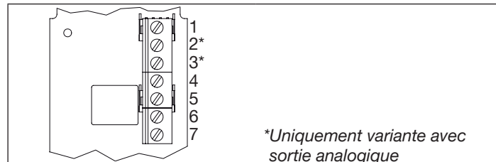
Fig. 11 : Bornes vissées
