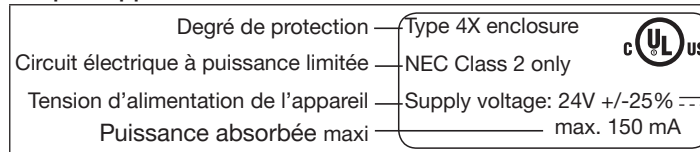
Fig. 4 : Plaque supplémentaire UL (exemple)
