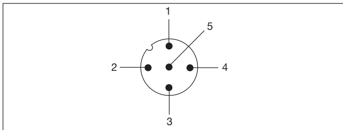
Fig. 14 : Affectation des raccordements, Port Class B
