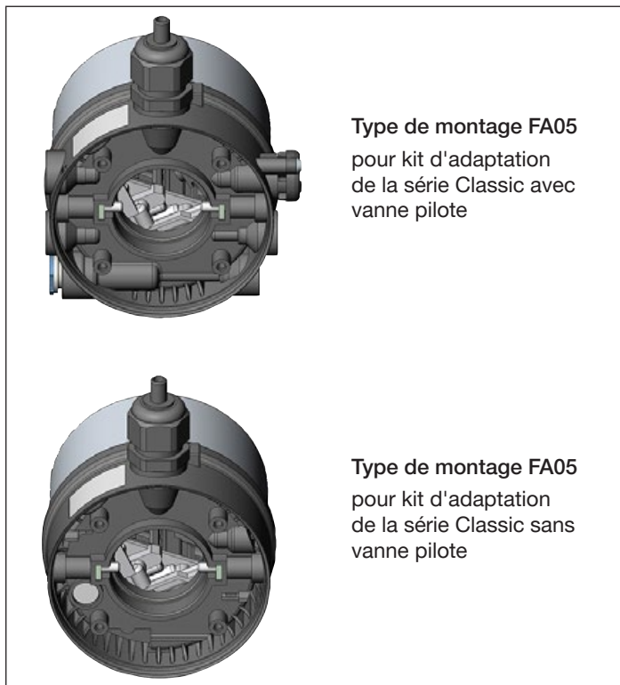
Fig. 7 : Type de montage FA05
