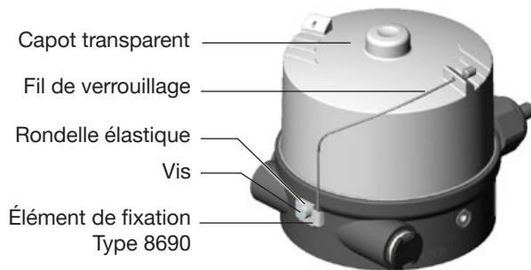
Fig. 4 : Montage du fil de verrouillage
