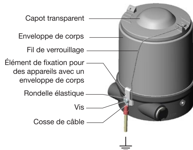
Fig. 5 : Montage du fil de verrouillage et mise à la terre
