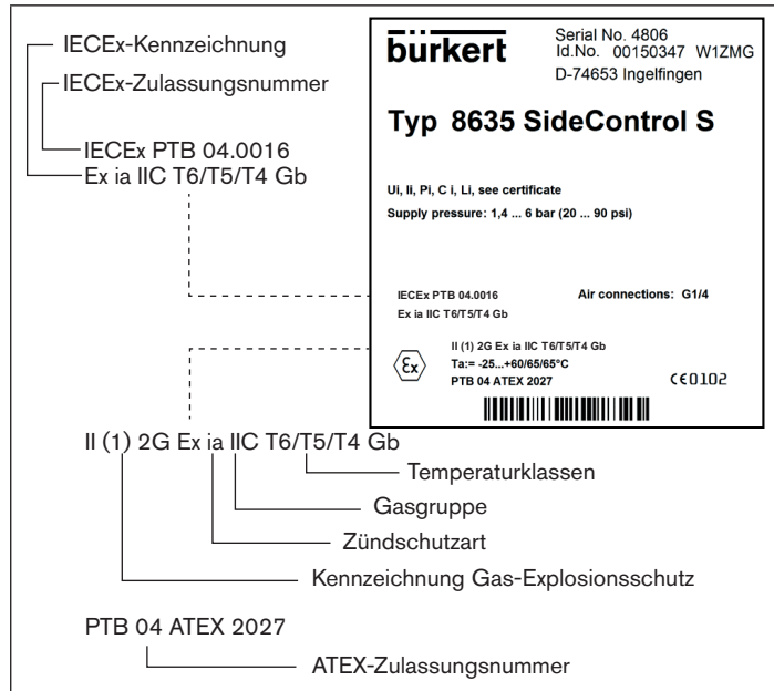
Bild 1: Typschild für Ex-Bereich
