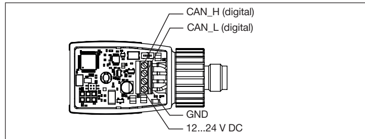
Bild 2: Anschluss Klemmleiste
