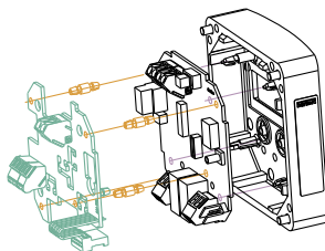
With relays / Avec relais / Mit Relais
