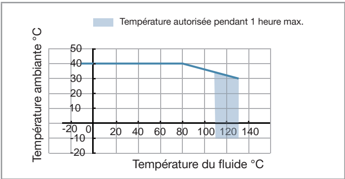
Fig. 2 : Température du fluide en fonction de la température ambiante pour un produit ATEX ou IECEx
