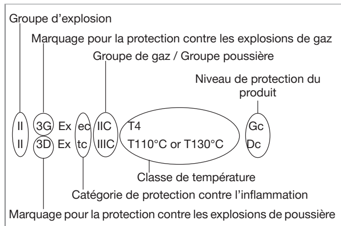
Fig. 1 : Marquage supplémentaire pour zones Ex
