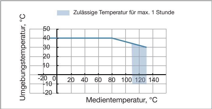
Abb. 2: Medientemperatur abhängig von der Umgebungstemperatur für ein ATEX- oder IECEX-Produkt
