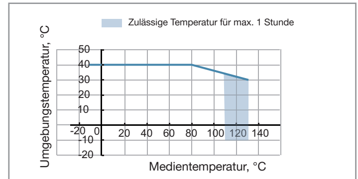
Abb. 2: Medientemperatur abhängig von der Umgebungstemperatur für ein ATEX-Produkt
