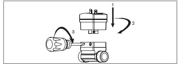
Fig. 1 : Montage du SE30 HT sur le raccord-captteur S030 HT
