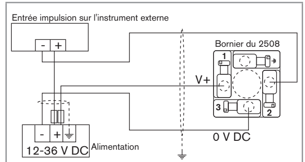
Fig. 4 : Câblage en NPN de la version avec sorties impulsion
