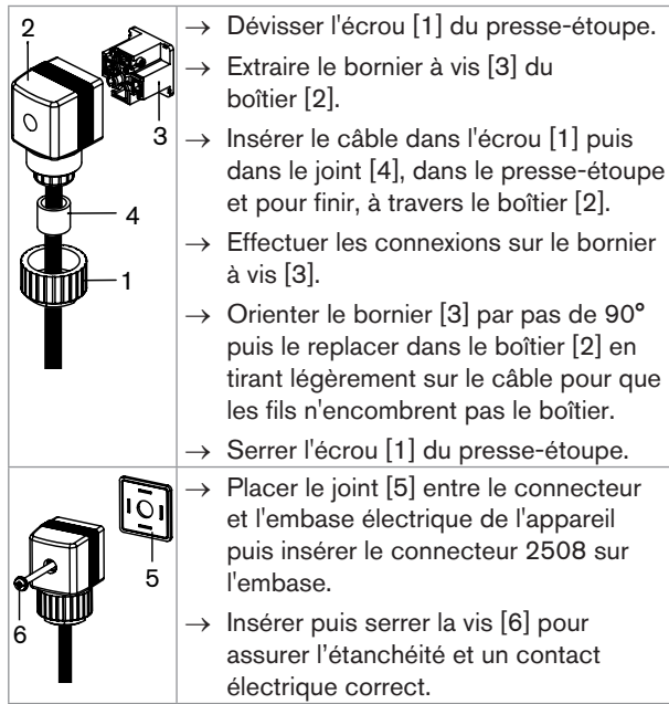
Fig. 2 : Assemblage du connecteur femelle type 2508 (fourni)
