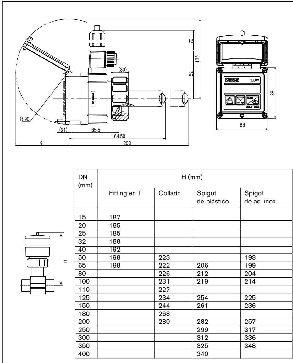
Fig. 2.1 Dimensiones del caudalímetro compacto 8025
