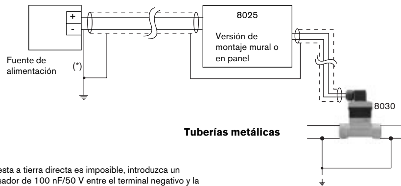
Esquema de equipotencialidad de un caudalímetro en versión independiente:
