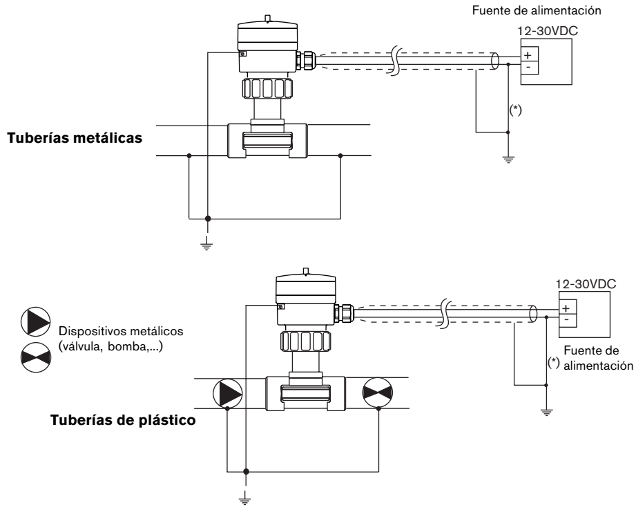
Esquema de equipotencialidad de un caudalímetro en versión compacta:
