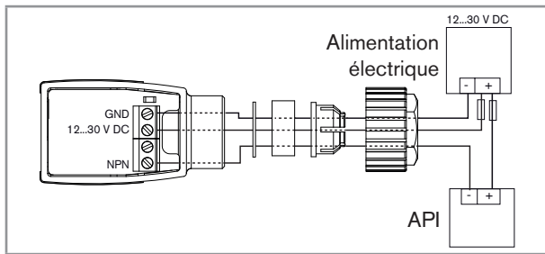
Fig. 4 : Appareil avec presse-étoupe – raccordement NPN de la sortie transistor
