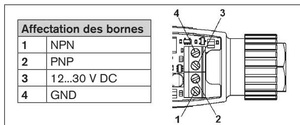
Fig. 2 : Affectation des bornes d'une variante d'appareil avec presse-étoupe
