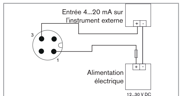
Fig. 7 : Appareil avec connecteur mâle M12 4 pôles – raccordement de la sortie courant
