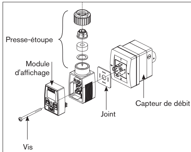
Fig. 10 : Monter l'appareil sur un capteur (Exemple d'un appareil avec presse-étoupe et module d'affichage, monté sur un capteur de type SE30)
