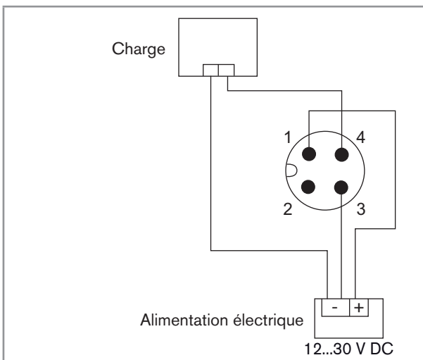
Fig. 9 : Appareil avec connecteur mâle M12 4 pôles – raccordement PNP de la sortie transistor
