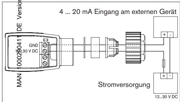
Bild 3: Gerät mit Kabelverschraubung – Anschluss des Stromausgangs
