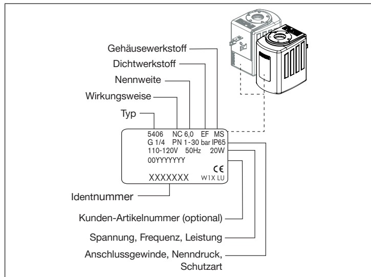
Bild 1: Lage und Beschreibung des Typenschildes
