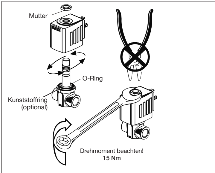
Bild 5: Spulenmontage
