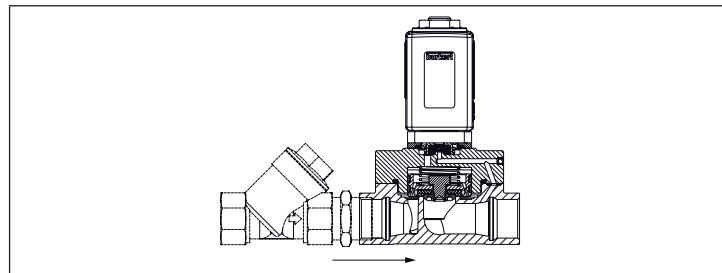
Bild 3: Einbau des Schmutzfilters
