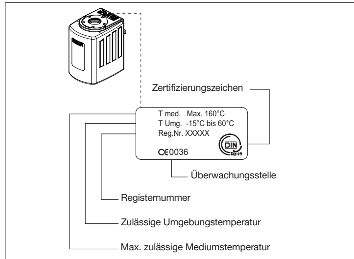
Bild 2: Lage und Beschreibung des Zusatzschildes
