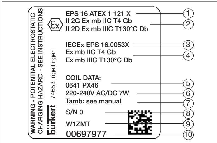
Bild 1: Beschreibung des Typschilds für Ex-Bereich (Beispiel)
