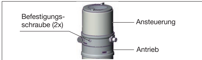
Bild 3: Ansteuerung demontieren
