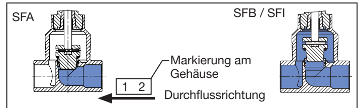
Bild 1: Anströmung unter Sitz (Ruhe auf/zu, gegen Medium schließend)
