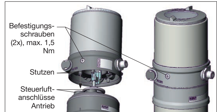
Bild 7: Montage Ansteuerung
