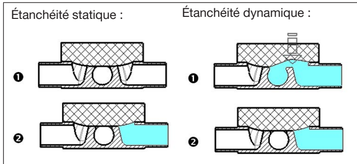
Fig. 1 : Étanchéité statique et dynamique
