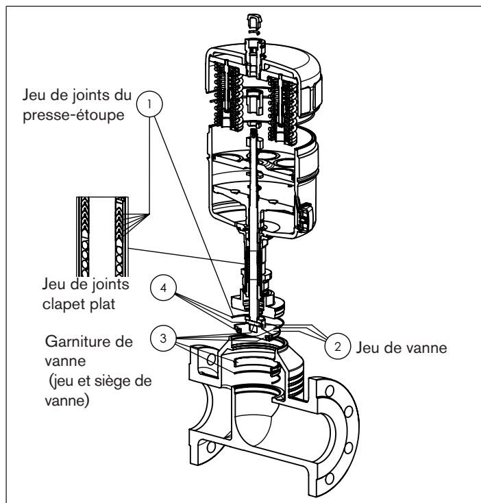
Figure 8 : Vue d'ensemble des jeux de pièces de rechange
