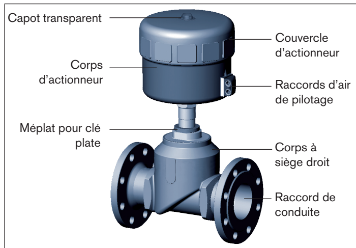
Figure 1 : Vanne à siège droit type 2012, structure et description
