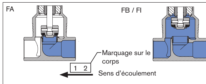
Figure 2 : Arrivée du fluide sous le siège (fermeture de la vanne contre le sens du flux de fluide)
