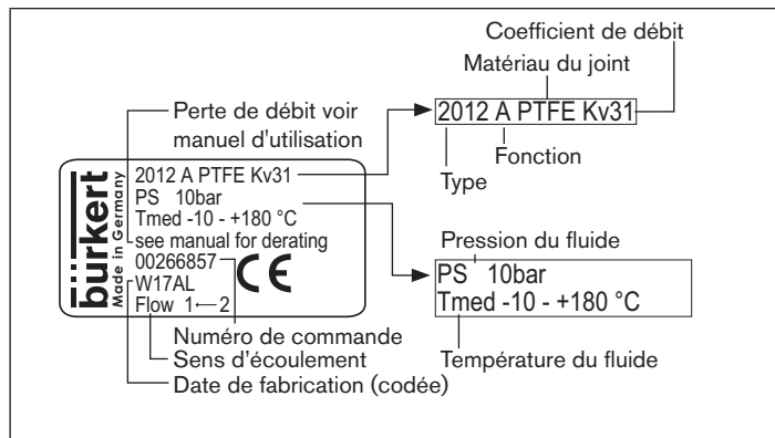
Figure 4 : Description de l'étiquette d'identification :
