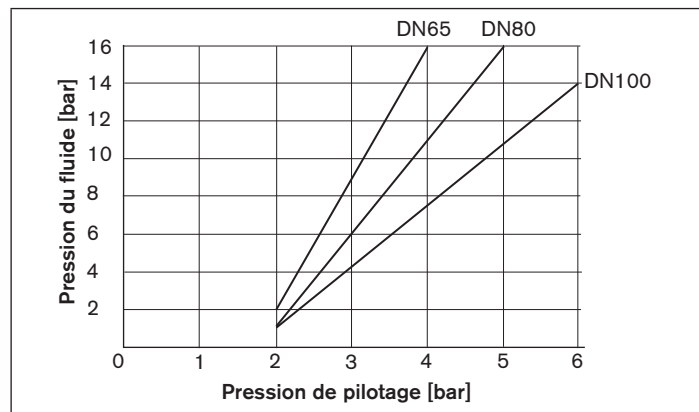
Figure 5 : Diagramme de pression, fonctions B et I, arrivée du fluide sous le siège
