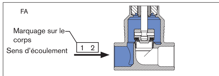
Figure 3 : Arrivée du fluide au-dessus du siège (fermeture avec le fluide)
