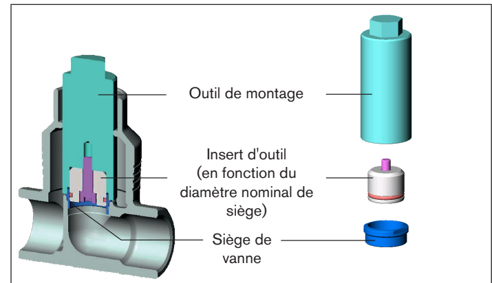
Figure 7 : Remplacement du siège de vanne
