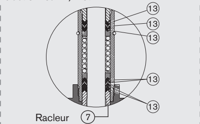
Presse-étoupe des vannes avec tailles d'actionneur D, E et F
