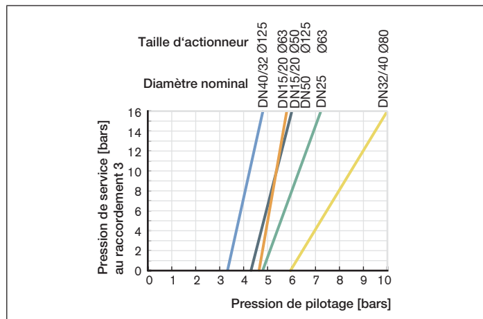
Fig. 4 : Diagramme de pression de pilotage (FA, sens du débit 3→2)
